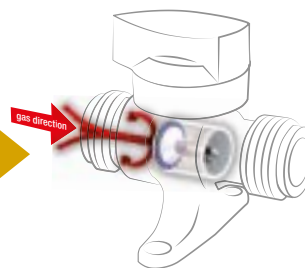
Coupure automatique de l'arrivée du Gaz due à l'excès de débit aval
